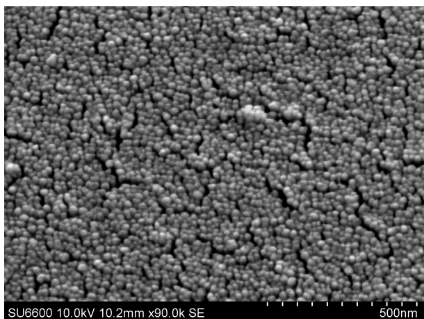
Фото 1: поверхность AFM® (500 nm)
