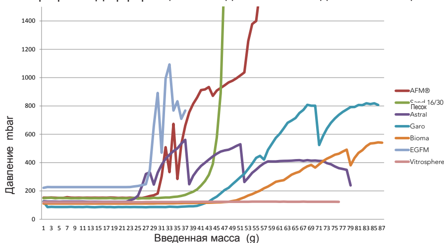
График 2: Дифференциальное давление и введенные частицы
