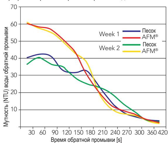
График 4: Кривые обратной промывки для песка и AFM®
