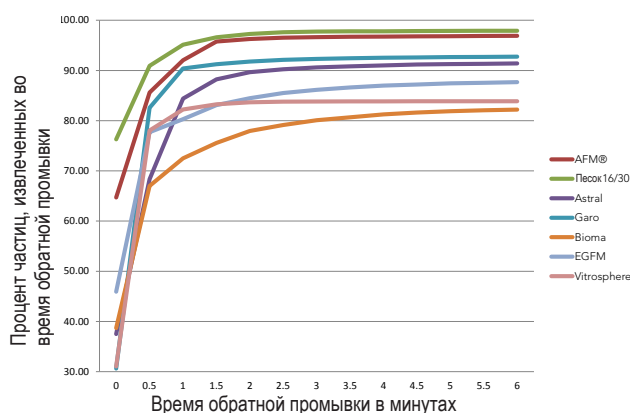
График 3: Эффективность обратной промывки
