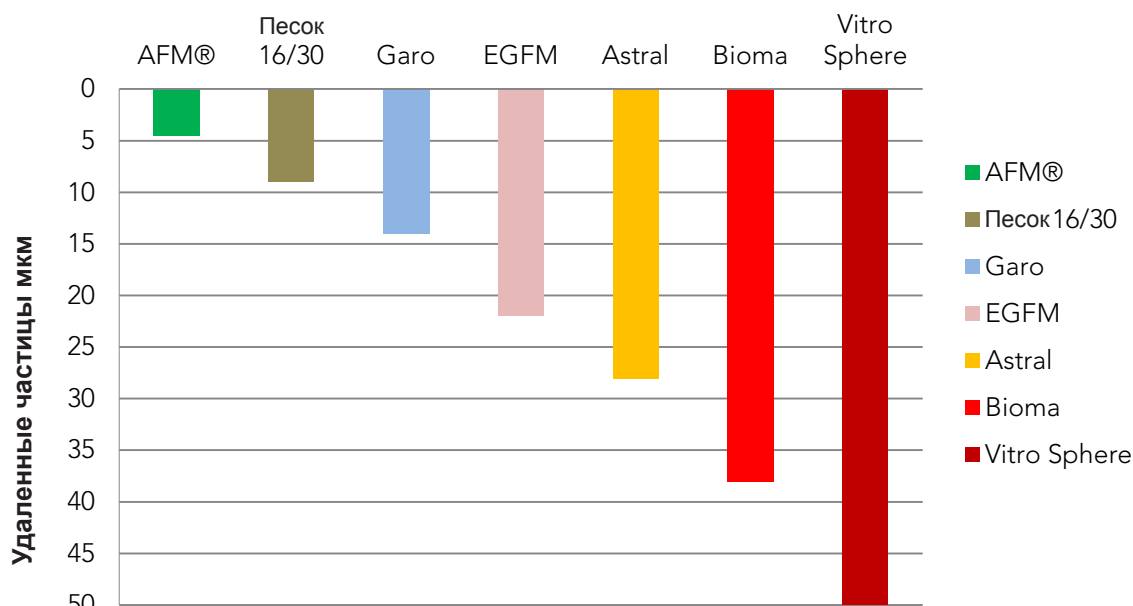
График 1: мельчайшие частицы, удаленные на 80 % при производительности 20 м/ч и без флокуляции
